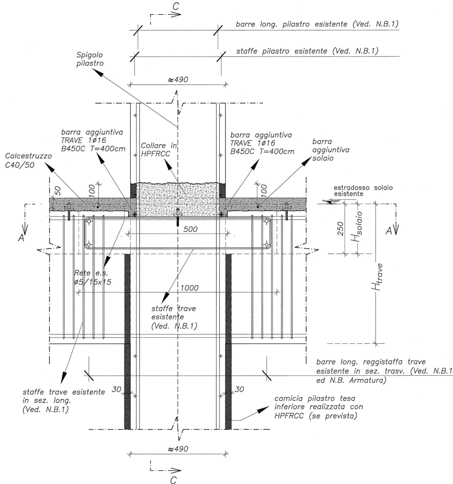
SEZIONE B-B VERTICALE 1:20
