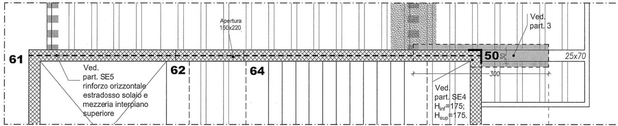
sezione scala 1:20
