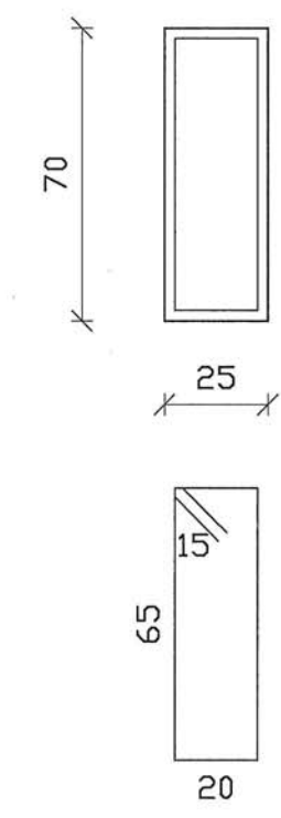
sezione scala 1:20
