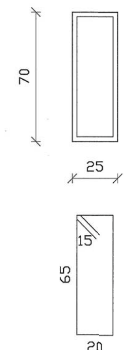
sezione scala 1:20
