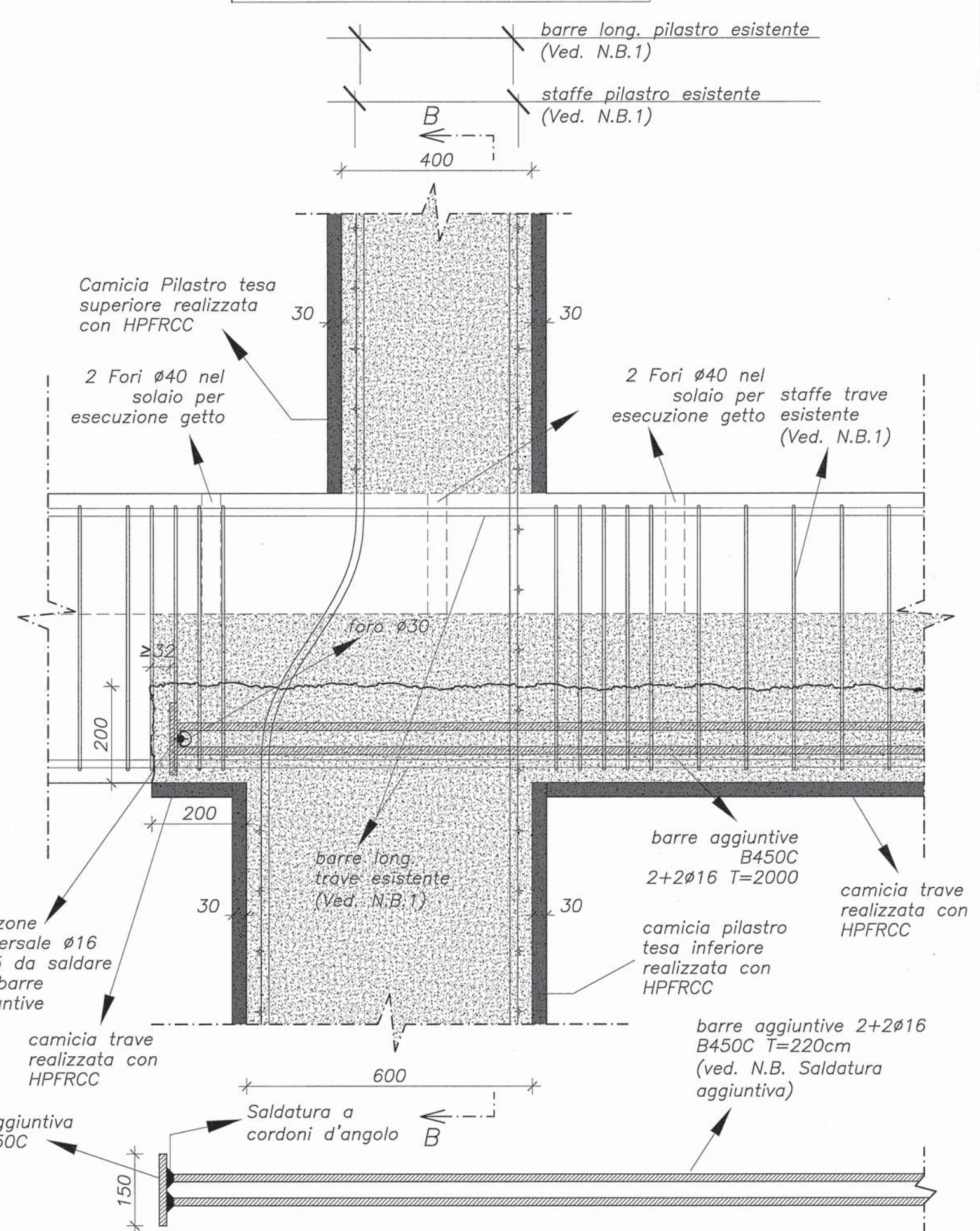
SEZIONE C-C VERTICALE 1:20
