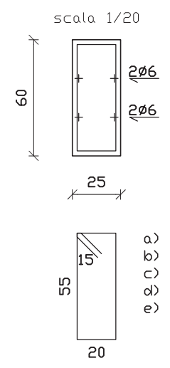
sezione scala
