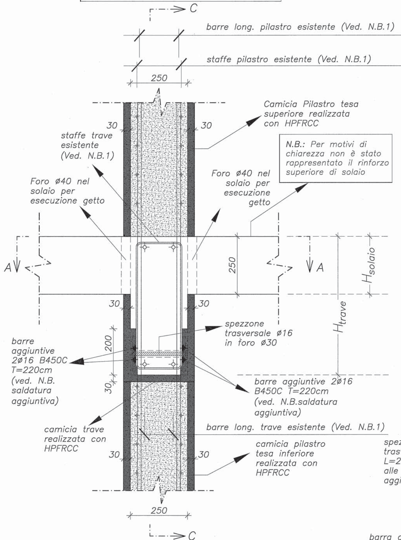
SEZIONE B-B VERTICALE 1:20
